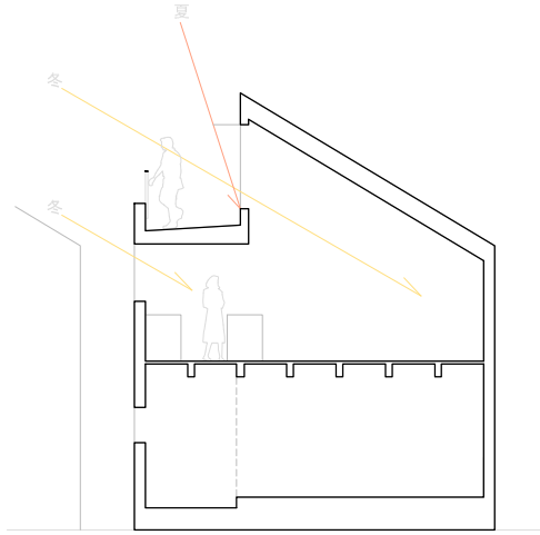
南-北 断面図
