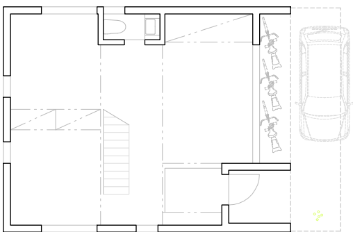
1階平面図
